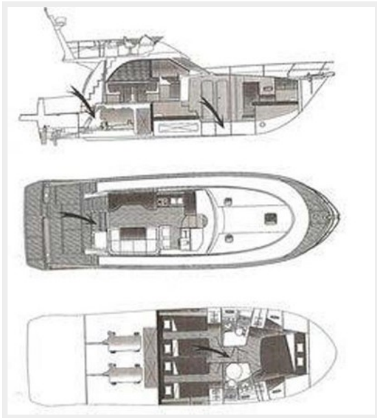
Beneteau Antares 45 - layout
