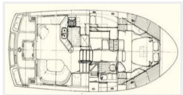
40' Nordhavn layout2
