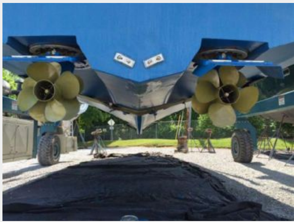
Fresh Bottom Paint & New Zincs 6/10/2015
