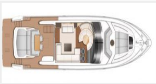
s72-layout-main-deck
