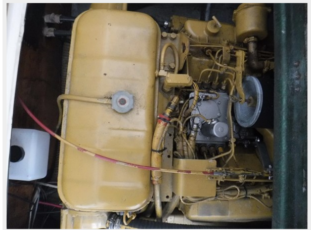
14 Cat 3208 Stbd
