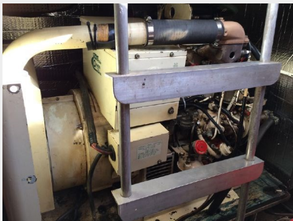
Genset
