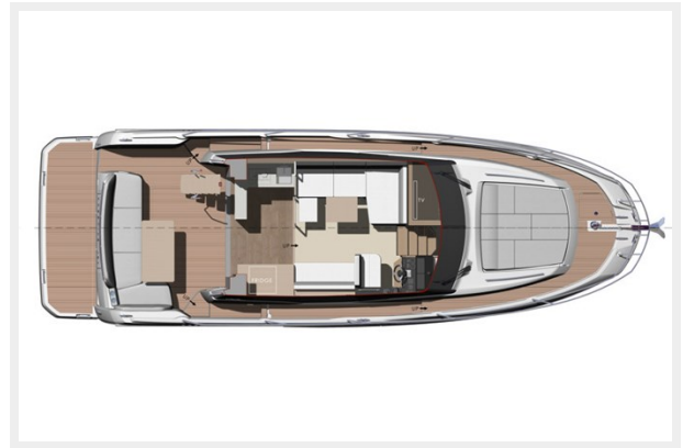
PRESTIGE-420---Main-deck--800px
