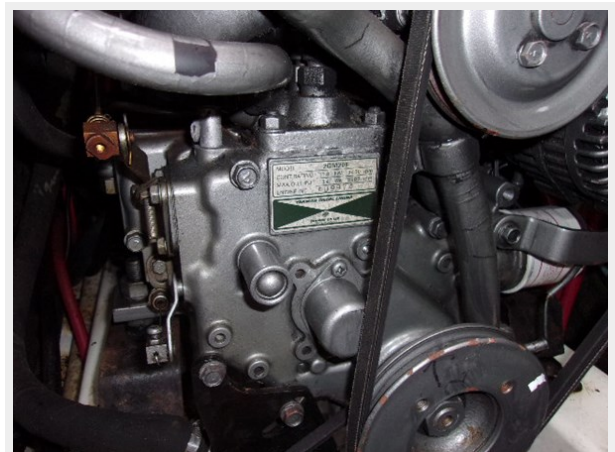
2004 Oceanis 311 Beneteau 58
