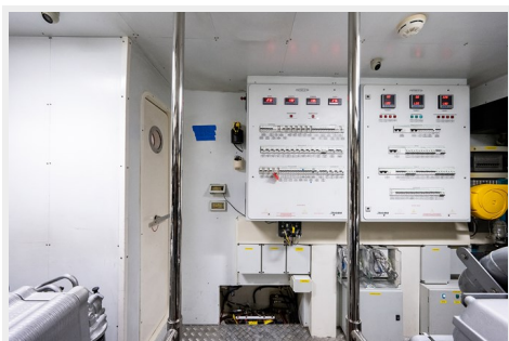
92_pershing_adiamo_engine_room14
