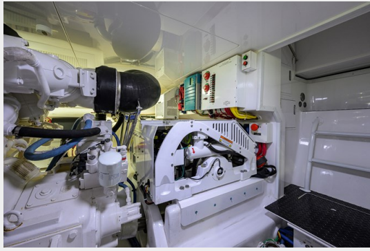
52_viking_mia_novia_engine_room_03
