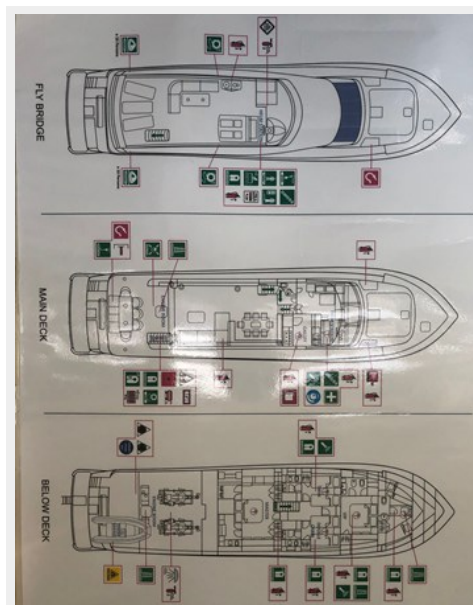
M.Y. Ocean Delta 11 - GA
