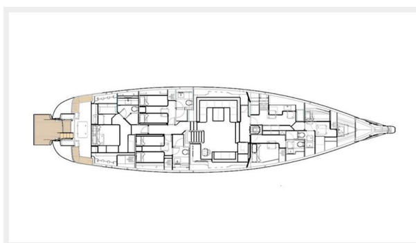
Enso Layout
