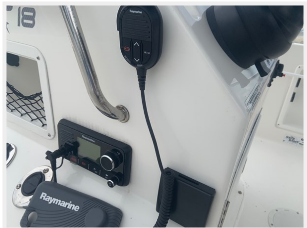
05.vhf
