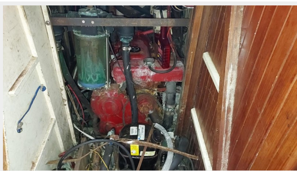
46_2798794_
