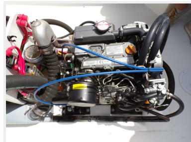
54_2800129_miss_baker_2017_ranger_tugs_r_21ec_yanmar_side_view
