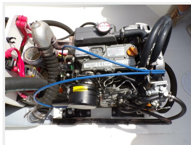
54_2800129_miss_baker_2017_ranger_tugs_r_21ec_yanmar_side_view
