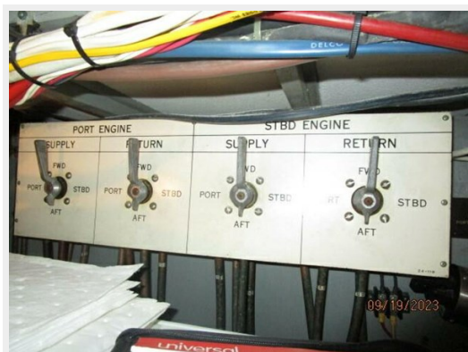
49_2803602_42_hatteras_fuel_manifold
